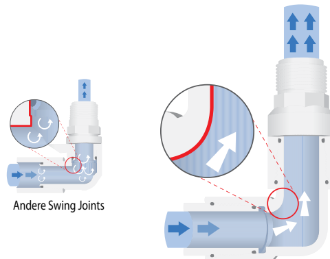
Rain Bird TSJ Swing Joints Hydraulisch optimiertes Design Minimale Druckverluste
