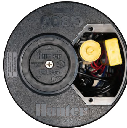
G885 Rotor TTS z układem dekodującym w głowicy
