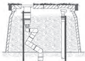
PRZEKRÓJ
