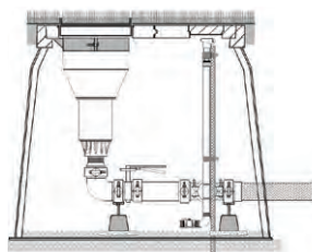
PRZEKRÓJ
