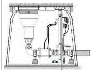
PRZEKRÓJ
