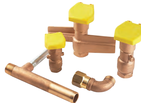
Szybkozłącza
