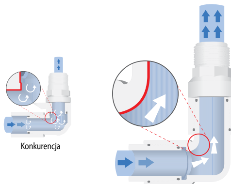
Nowatorski projekt kolanka przegubowego złącza Rain Bird TSJ Znacznie redukuje straty ciśnienia
